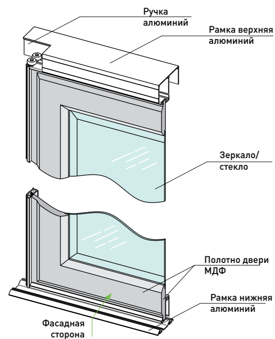
Схема односторонней двери
